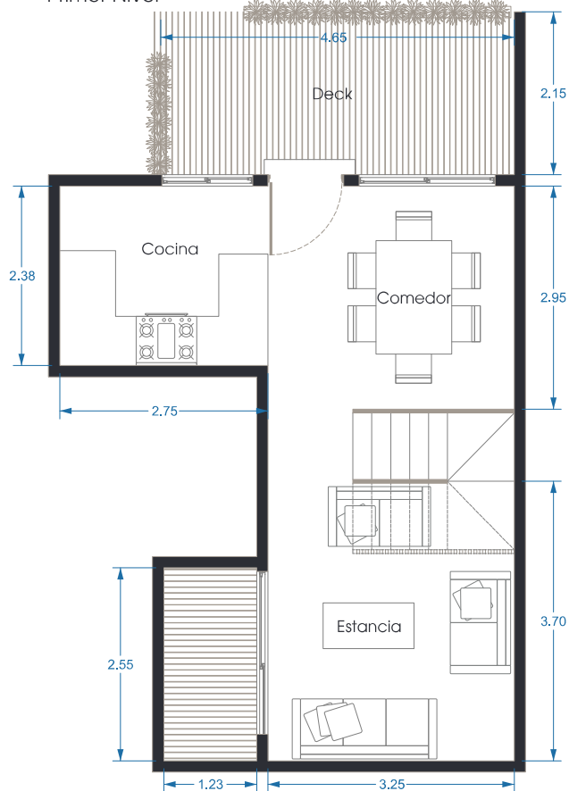
Planta Baja
