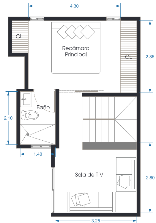
Segundo Nivel
