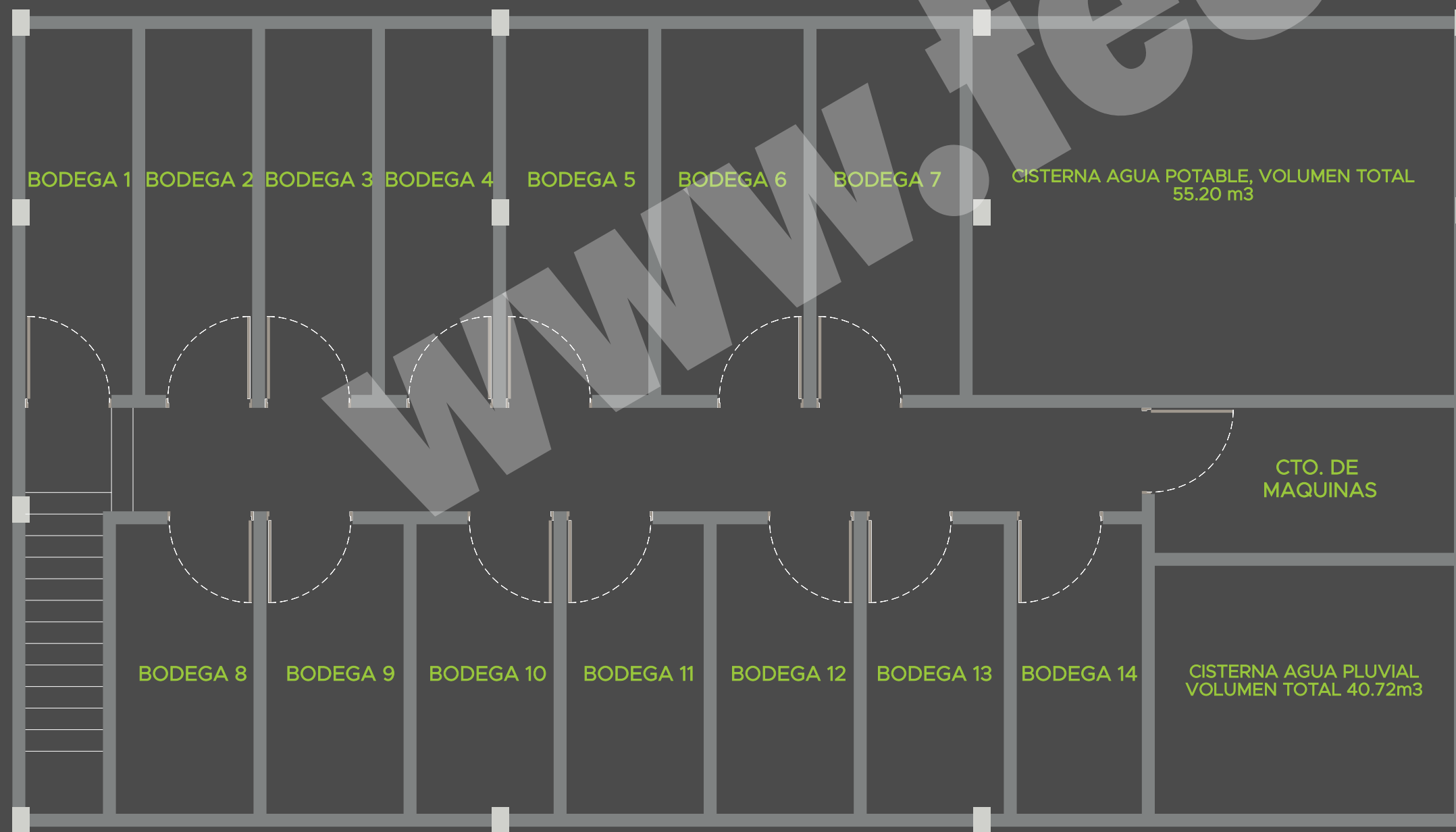
Planta Cisternas
