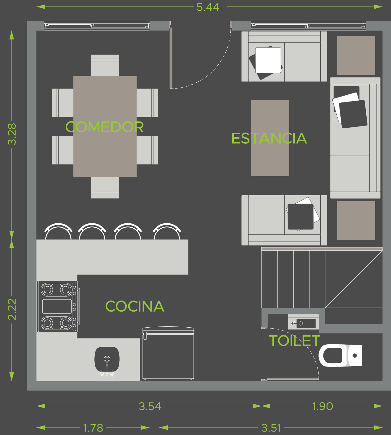
Planta Baja
